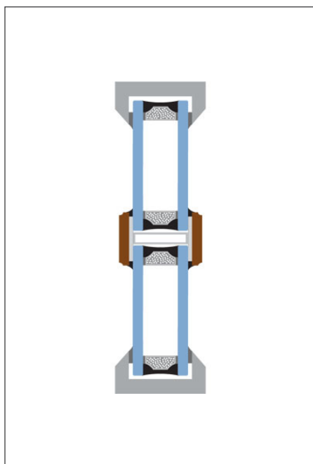
Glasteilende Sprosse
