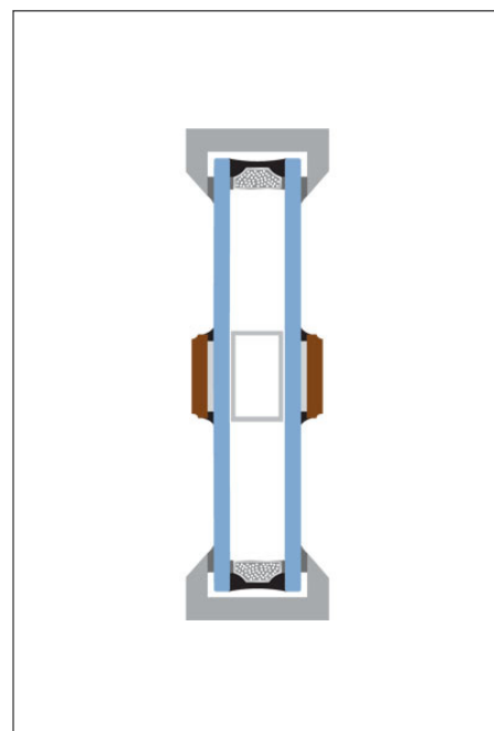
Wiener Sprosse
