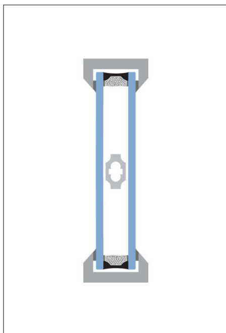
Innenliegende Dekosprosse
